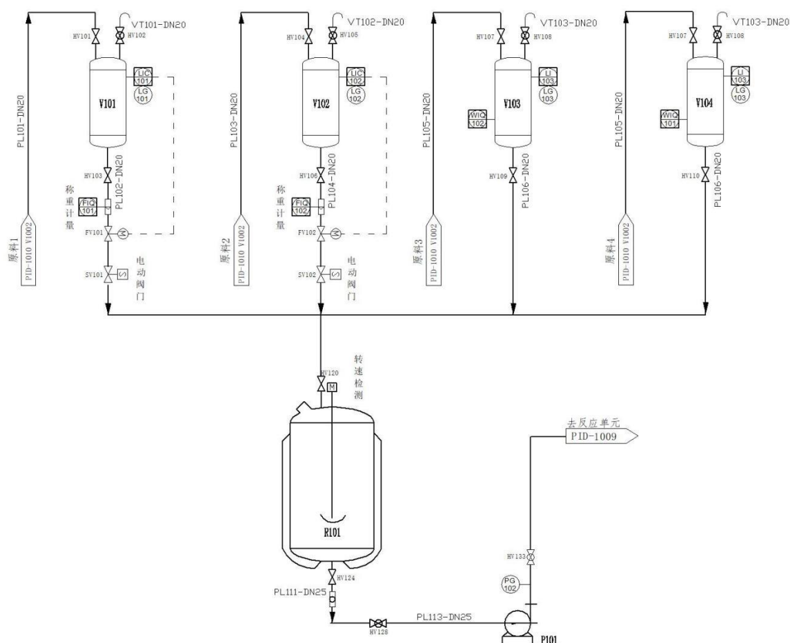
图 2 产品柔性化配料系统流程图(仅供参考)
