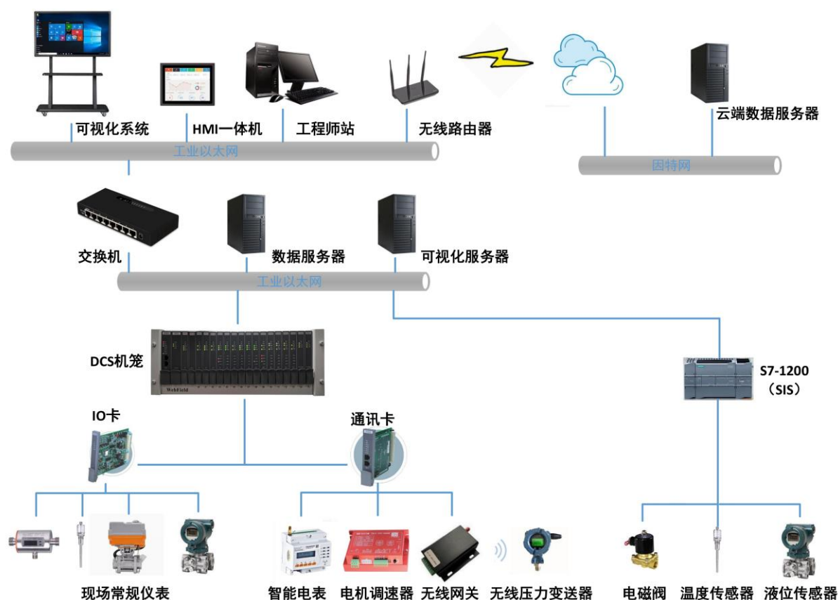
图 6 网络拓扑图(仅供参考)
