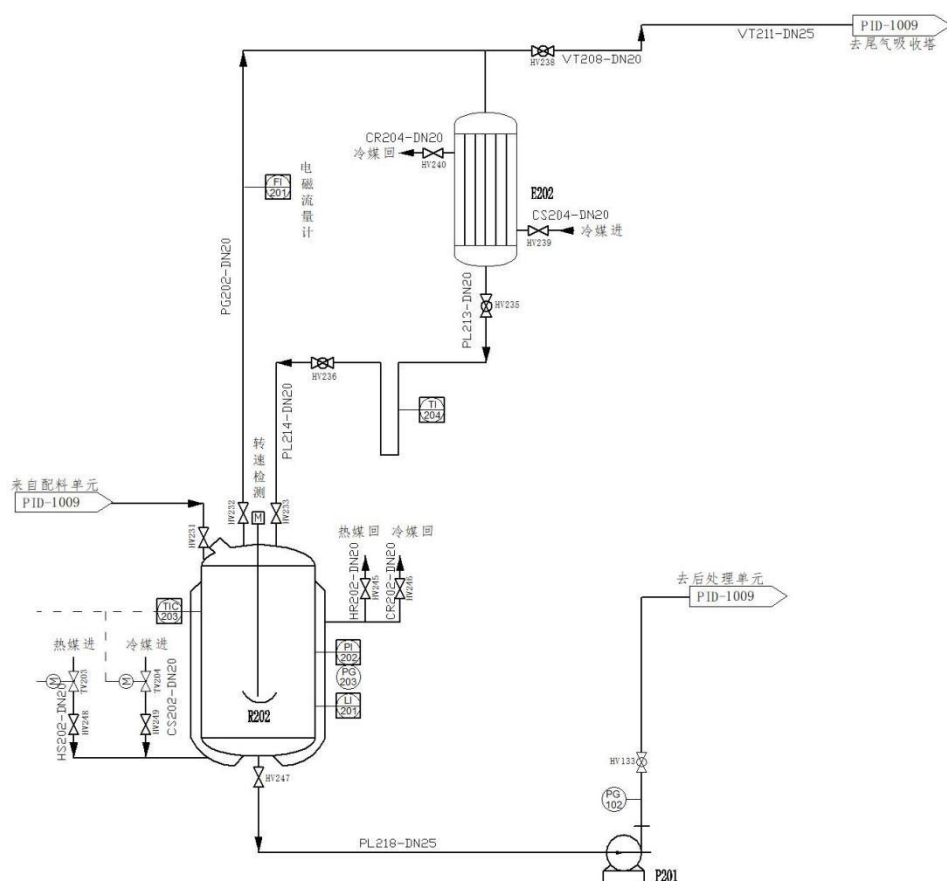
图 3 产品柔性化深加工系统流程图(仅供参考)
